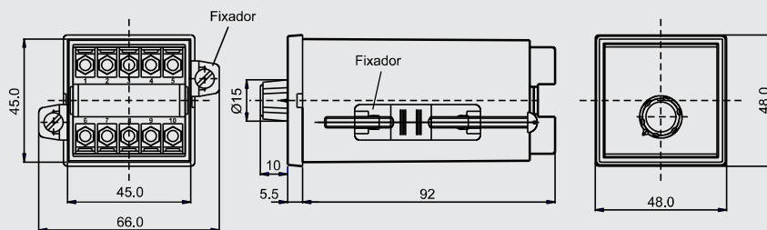
Caixa 48x48mm 10 terminais
