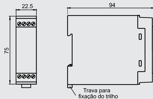
Caixa 22,5x75mm p/ 8 terminais
