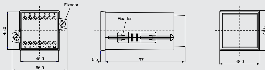
Caixa 48x48mm 14 terminais
