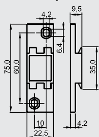
Fixador DIN sobrepor
