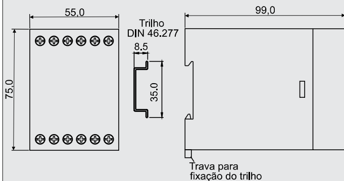
Caixa 55x75mm 12 terminais
