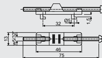
Fixador p/ painel
