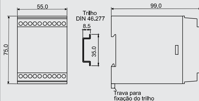
Caixa 55x75mm p/ 20 terminais
