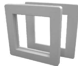
Adaptador ABS p/ substituir aparelho c/ furação 72 por 48mm Cinza - 1310-60 Preto - 1310-61
